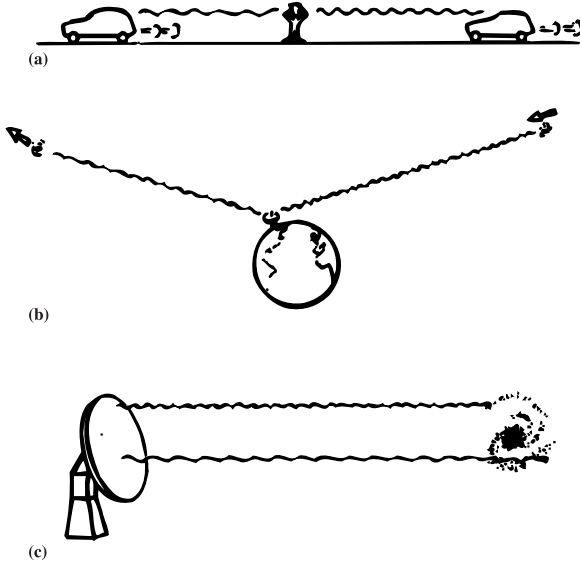
شكل (10- 2) إزاحة دوبلر.
